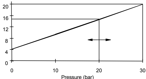
Output 4 ... 20 mA
