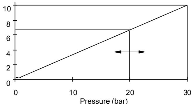
Output 0 ... 10 V
